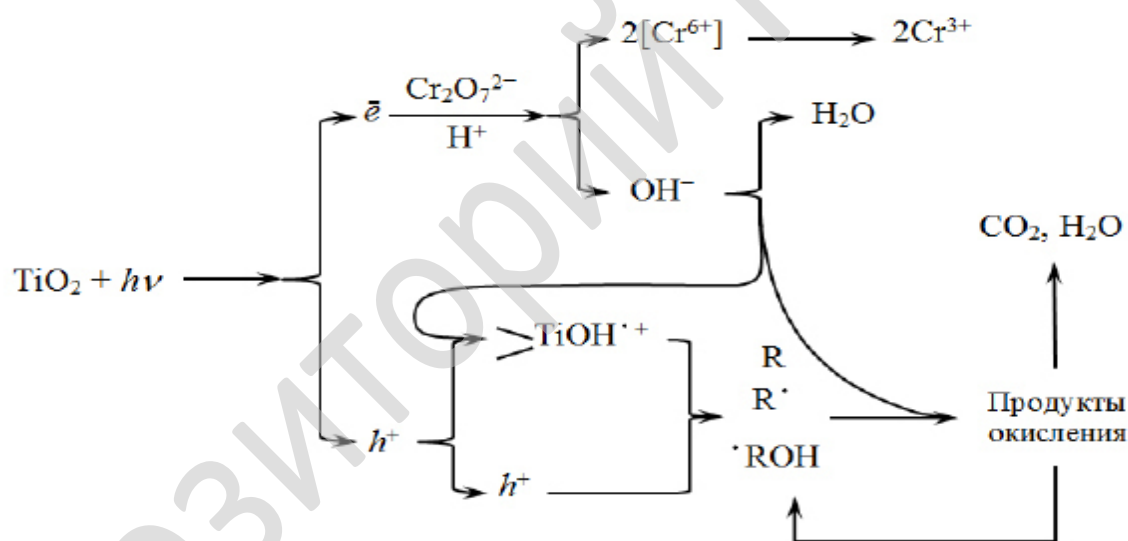
Рисунок 1. Схема фотокаталитической минерализации органических веществ с использованием дихромата калия в качестве поглотителя электронов
