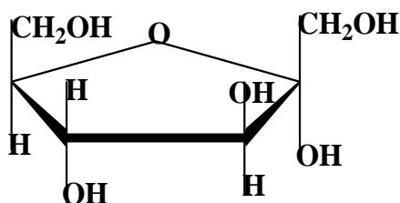
\alpha -D fructofuranose
