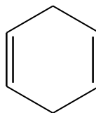
Cyclohexadiene-1,4
