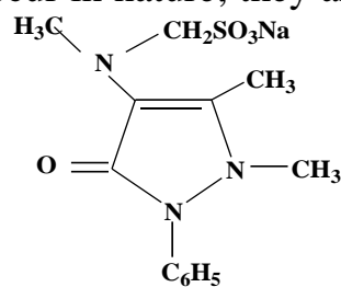
Analgine
