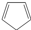
Cyclopentadiene-1,3
