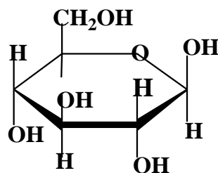
\beta -D- glucopyranose (64 %)
