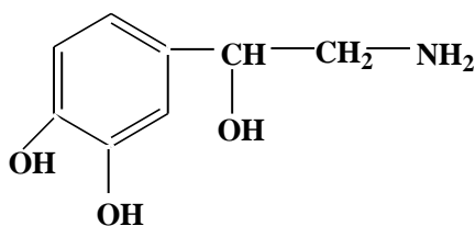
Noradrenalin
