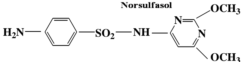
Norsulfasol
