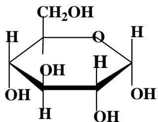
\alpha -D glucopyranose (36 %)
