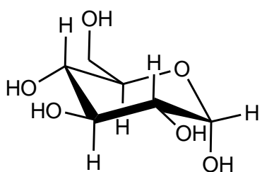
\alpha -D glucopyranose
