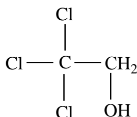
2,2,2-trichloroethanol-1
