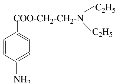
Novocain
