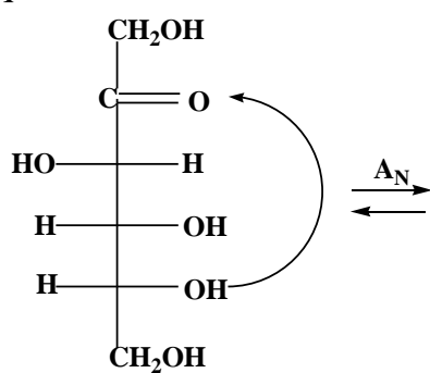
D-fructose
