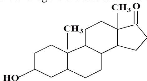
Androsterone
