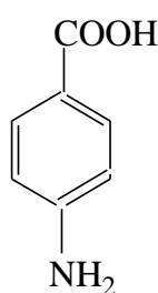
PABA
