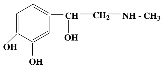
Adrenaline
