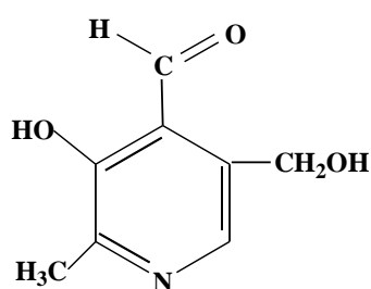
Pyridoxine (vitamin B 6 )
