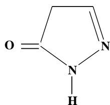
Pyrazalone-5
