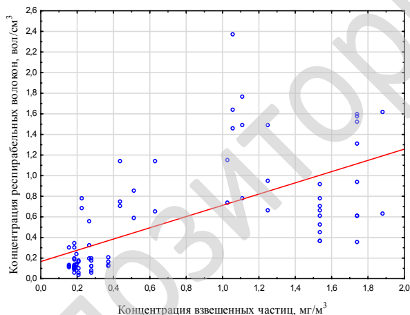
Рисунок 5. Линейная зависимость концентрации респирательных волокон хризотила от среднесменной концентрации массы взвешенных частиц
