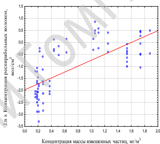
Рисунок 6. Модель нелинейной зависимости концентрации респирательных волокон хризотила от среднесменной концентрации массы взвешенных частиц
