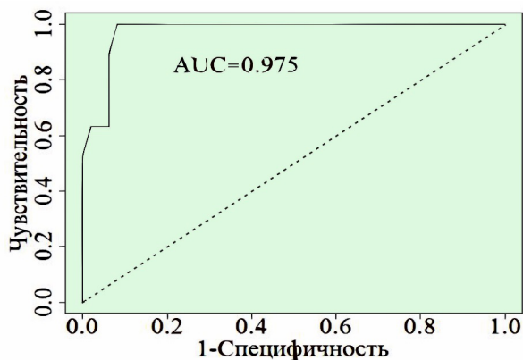
Рисунок 2. ROC-кривая модели
