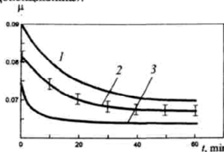
Рисунок 2 – Зависимость коэффициента трения в опоре трибометра от времени действия поля соленоида на смазочные слои аутосыворотки крови (подробности в тексте). Доверительные интервалы одинаковы для всех кривых
